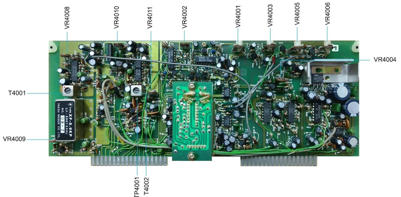
AF UNIT (PB-2252)
