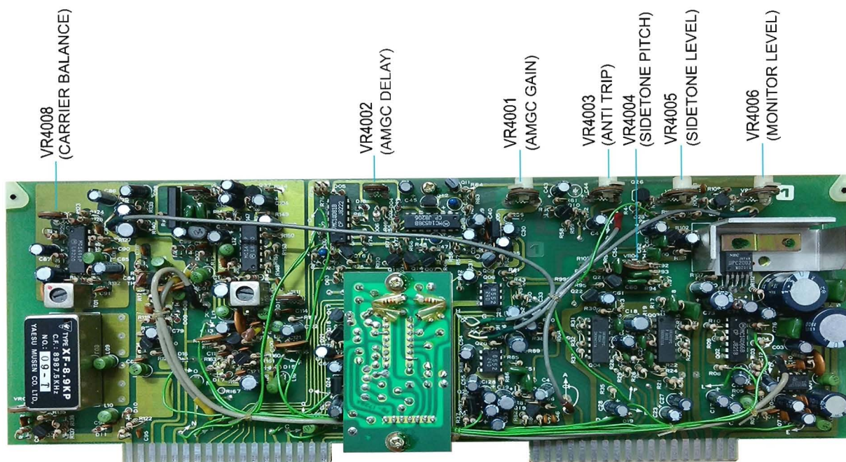
AF UNIT (PB-2252)
