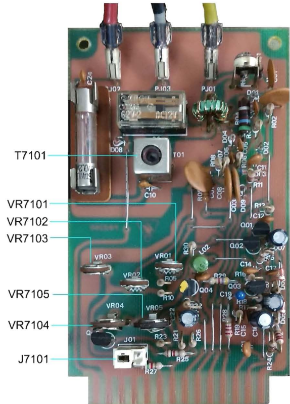
ALC UNIT (PB-2260)
