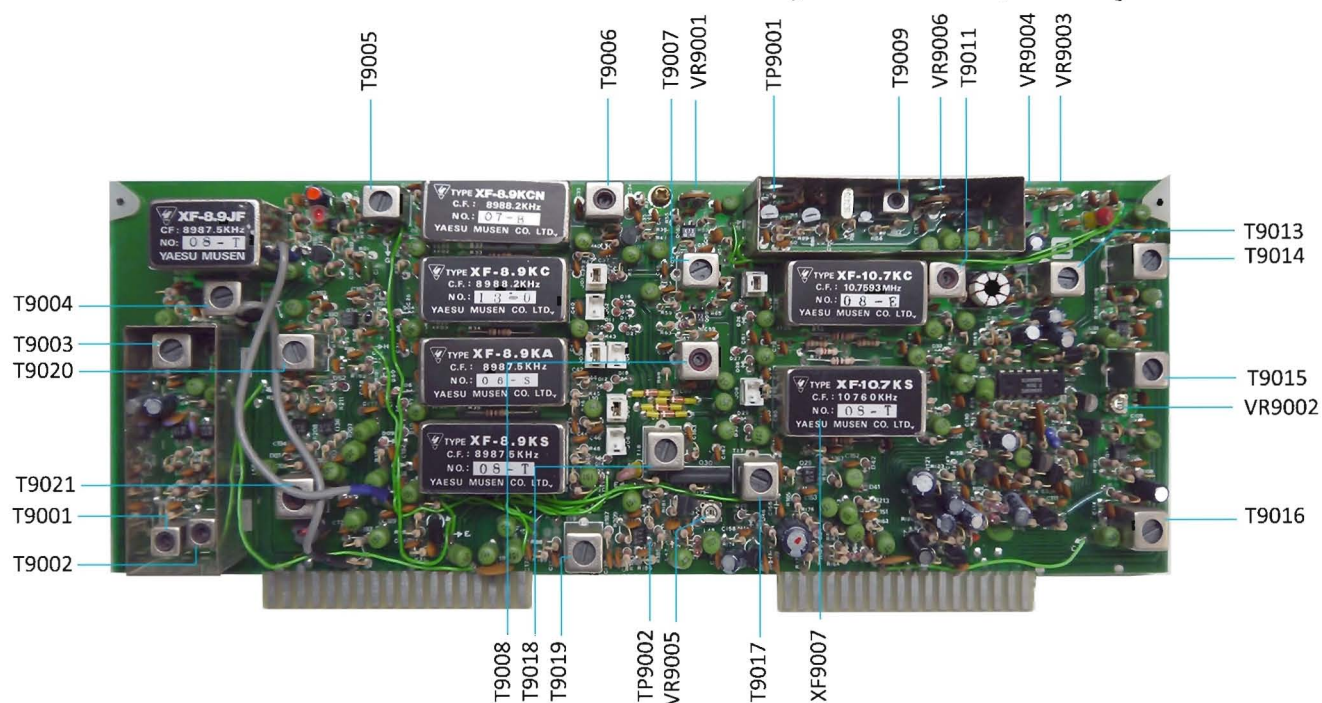
IF UNIT (PB-2255)
