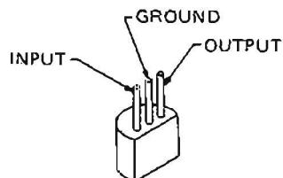
μPC78L08
